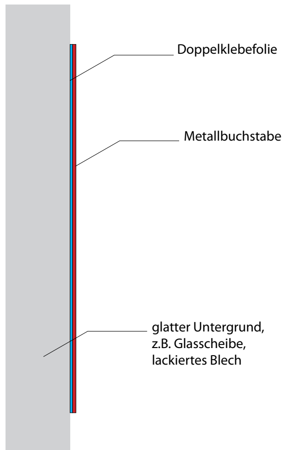
Befestigung durch Doppelklebefolie
