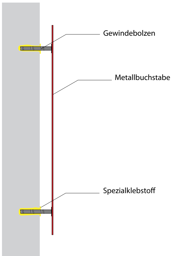
Befestigung durch Gewindebolzen
