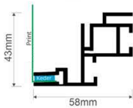
← → 58mm Bautiefe
