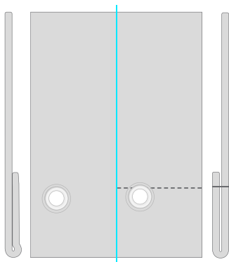
Saum, geschweisst oder genäht und geöst
