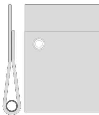
Hohlraum, geschweisst und geöst, z.B für Rundrohr
